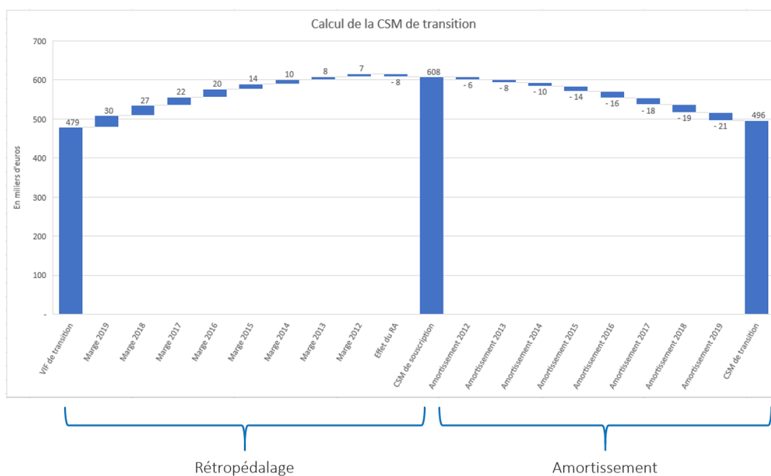
FIGURE A.14 – Méthode MRA - Enroulement de la CSM du produit Digital dans l'environnement de hausse des taux
