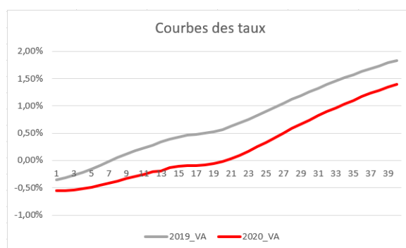
FIGURE 8.1 – Courbes des taux sans risques de l'EIOPA en 2019 et 2020
