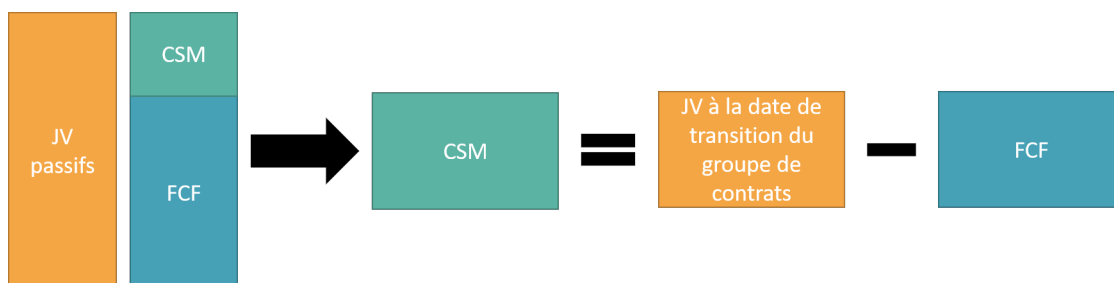
FIGURE 3.4 – La CSM selon l'approche FVA
