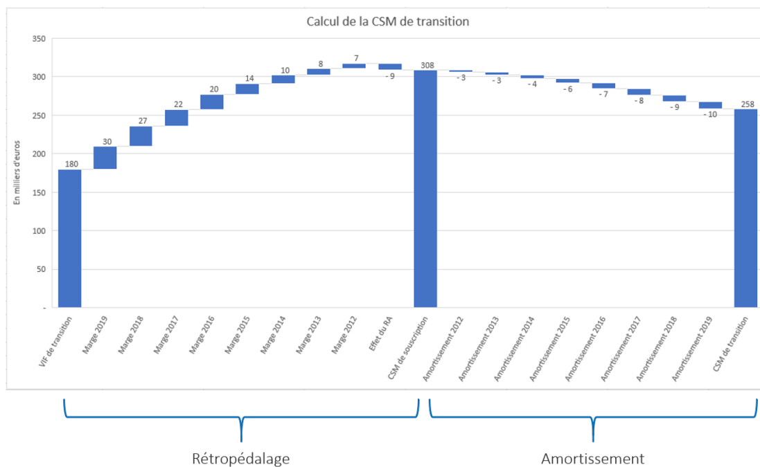
FIGURE A.22 – Méthode MRA - Enroulement de la CSM du produit Digital sans allocation de la RC la PVFP
