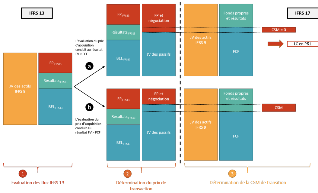
FIGURE 6.3 – Méthodologie proposée pour la FVA
