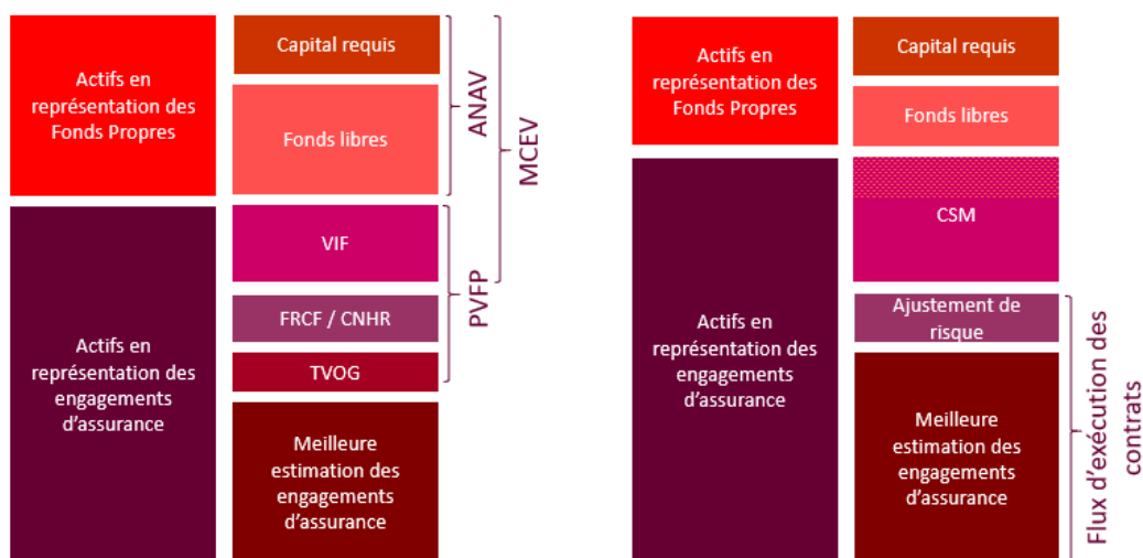
Référentiel MCEV
