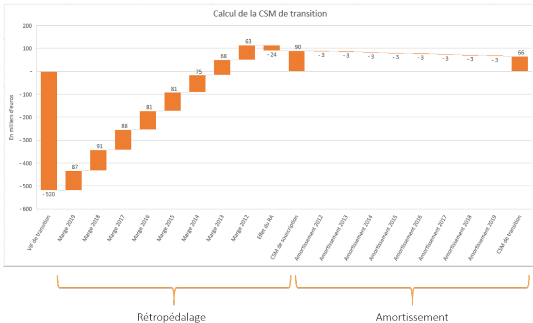
FIGURE A.5 – Méthode MRA - Enroulement de la CSM du produit Traditionnel dans le scénario de baisse des taux
