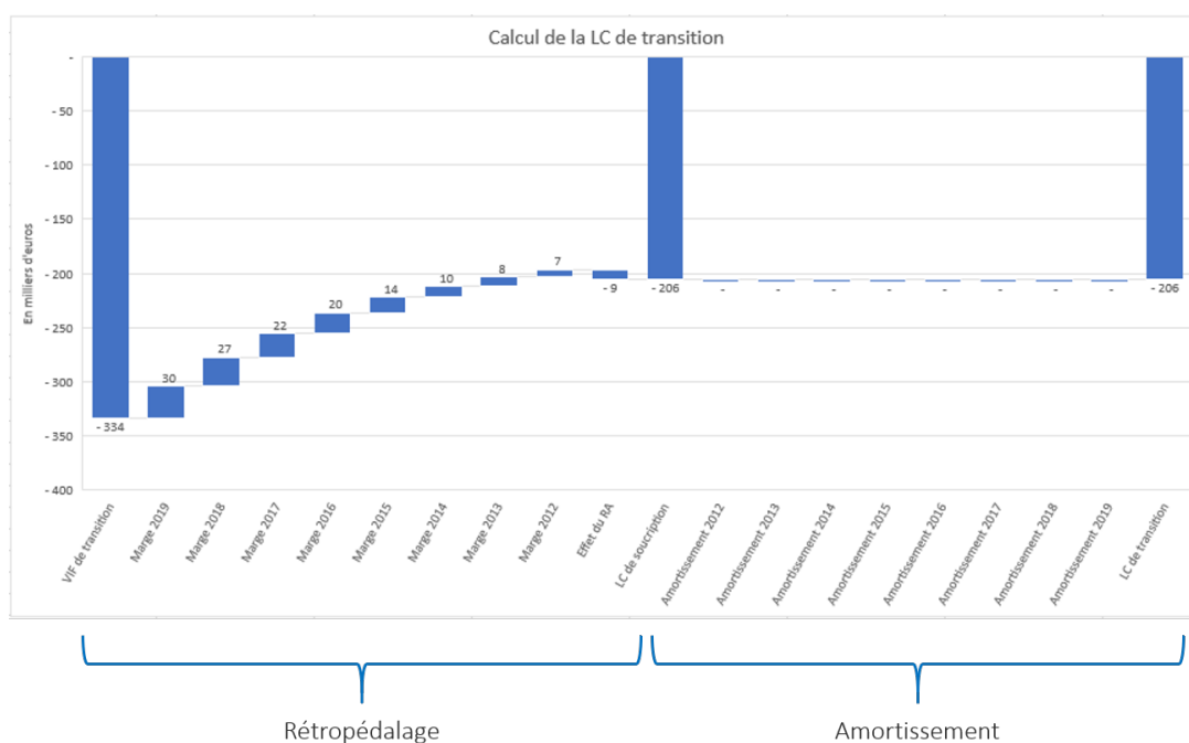
FIGURE A.6 – Méthode MRA - Rétropédalage de la LC du produit Digital dans le scénario de baisse des taux
